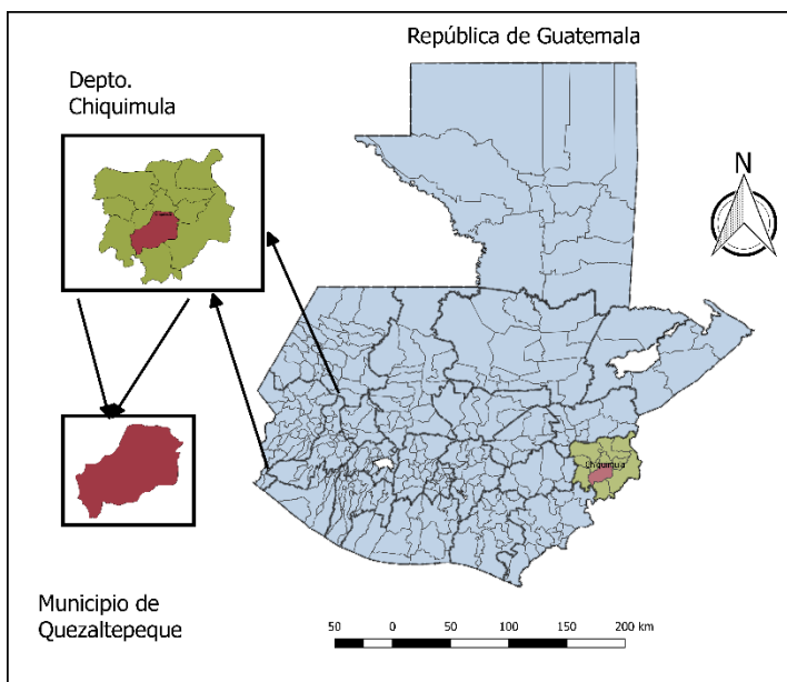
Mapa No. 1 Mapa de ubicación del municipio de Quezaltepeque, Chiquimula
